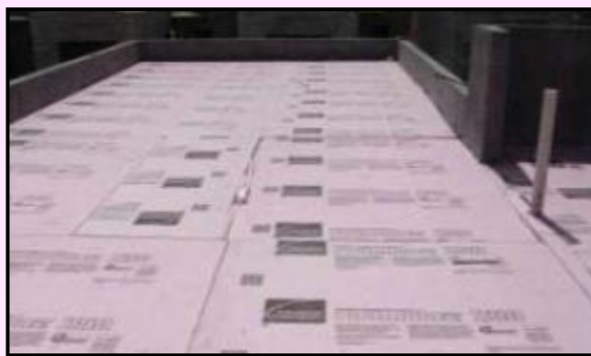
2) Cobrir toda a laje de concreto com o Foamular. Sem fixação requerida.
